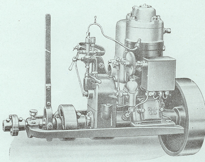
Marinmotor Typ BA 3, 4—5 hkr Urustning MB
