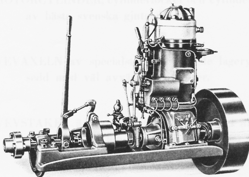
MARINMOTOR Typ A med utrustning F.
