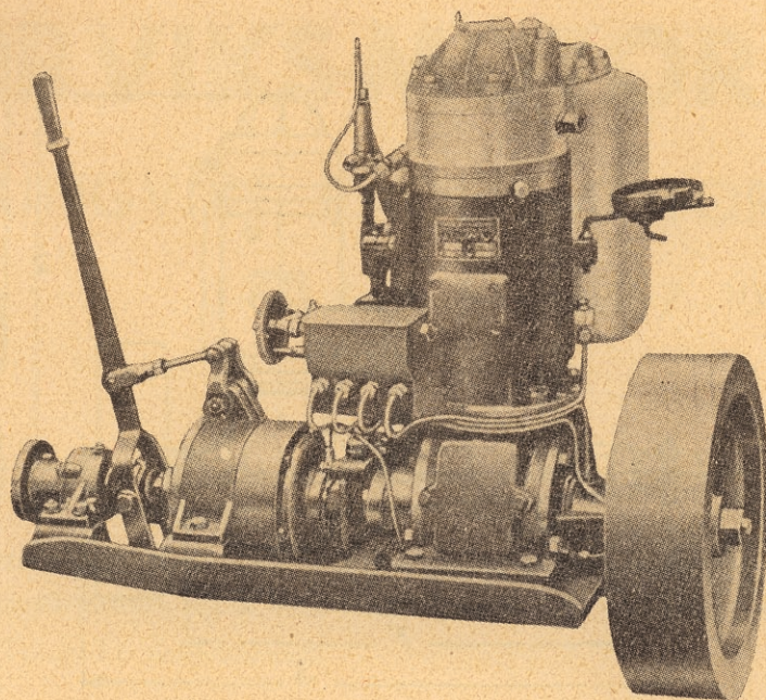
MARINMOTOR Typ A med utrustning F.
